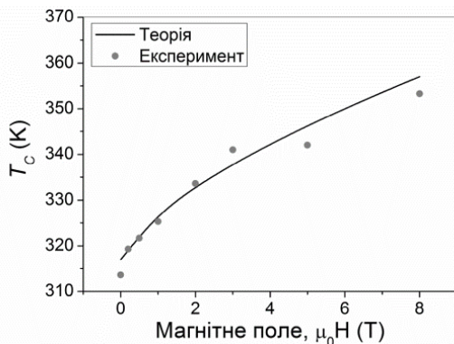
Рис. 2. Експериментальна та теоретична залежності температури Кюрі від величини магнітного поля [3].
