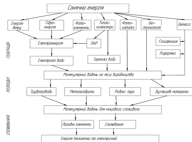
Рис. 2. Шляхи реалізації водневої енергетики
