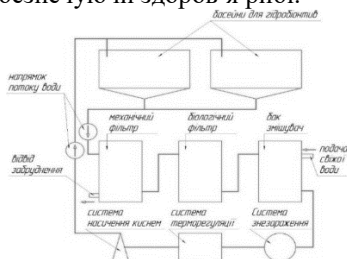
Рис. 1. Схема установки замкнутого водозабезпечення (УЗВ)
