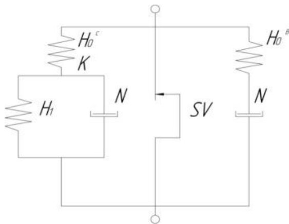
Рис. 4. Реологічна пружно-в'язка модель ґрунту
