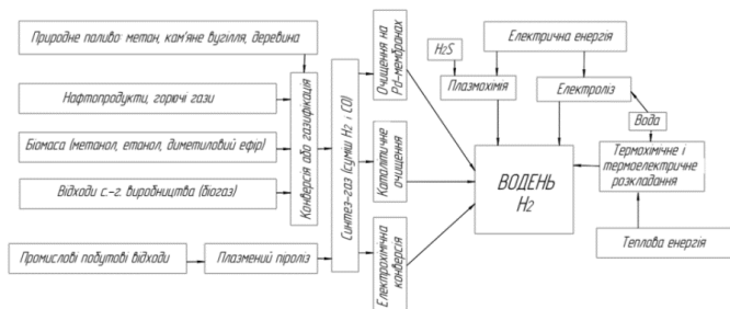
Рис. 1. Традиційні напрями отримання водню
