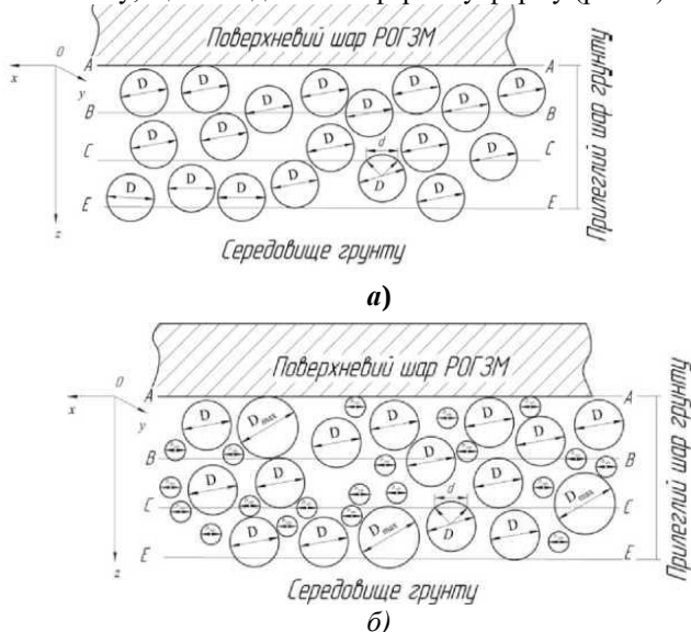
Рис. 3. Схема взаємодії поверхневого шару робочого органу з шаром ґрунту: а) монодисперсний шар ґрунту; б) полідисперсний шар ґрунту
